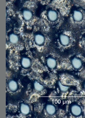
Edelstahlfolie mit lasergebohrten Löchern.
