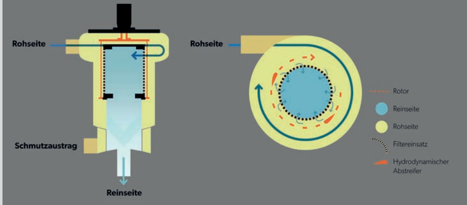
Funktionsprinzip des Zyklonfilters.
